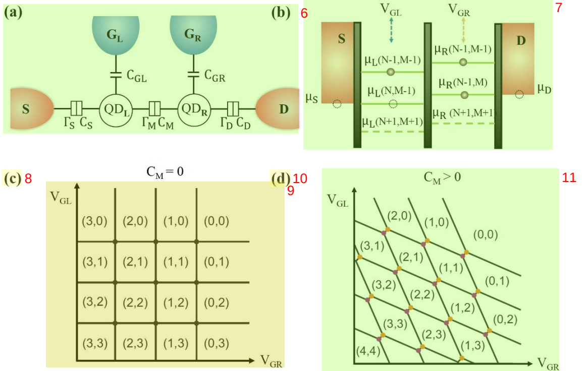
图 1.2(a) 双量子点电路模型示意图, 左边量子点 QD_L 和右边量子点 QD_R 通过 \Gamma_M 和 C_M 耦合。(b) 双量子点中电势 \mu_L 和 \mu_R 的示意图。(c) 零源漏偏压下左右两个量子点的耦合 C_M = 0 时双量子点的电荷稳定性相图。(d) 零源漏偏压下左右两个量子点的耦合 C_M > 0 时双量子点的电荷稳定性相图。
