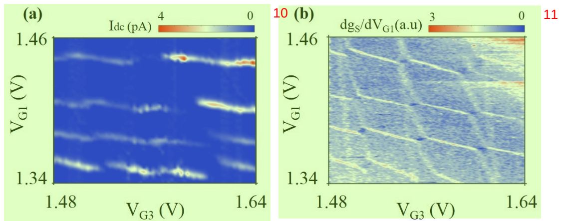
图 5.5(a) V_{SD} = 0.05 \text{ mV} , V_{G2} = 1.2 \text{ V} 时, 双量子点直流输运的稳定性相图。(b) 电荷感应器读取的微分电导相图。 12
