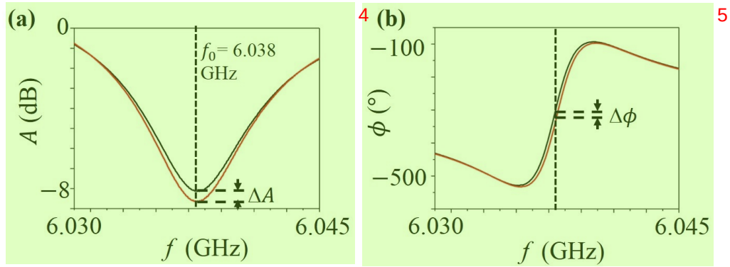
图 4.4 微波腔的幅值(a)和相位(b)随驱动频率演化的函数。黑色实线代表当量子点进入库伦阻塞区腔的信号，红色实线代表当量子点进入库伦共振区腔的信号。幅值和相位的变化分别用 \Delta A 和 \Delta \phi 表示，可以清楚地观测到。 6
