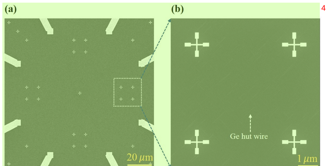
图 2.7 (a) 对应于图 2.6(a)中蓝色虚线方框区域内的一组大电极以及标记。(b) 包含 mark 以及纳米线的高分辨率图像，对应于(a)中白色虚线方框区域。
