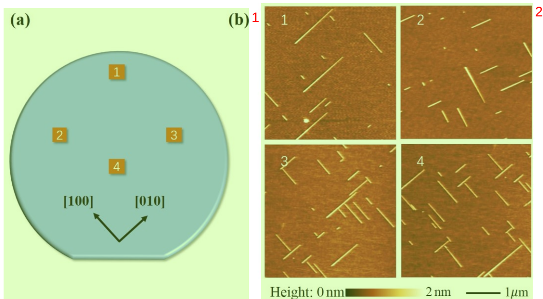
图 2.4 (a) 实验中所使用的四寸 Si 衬底基片示意图。(b) Ge 纳米线的 AFM 图，对应于图(a)中 4 个区域。
