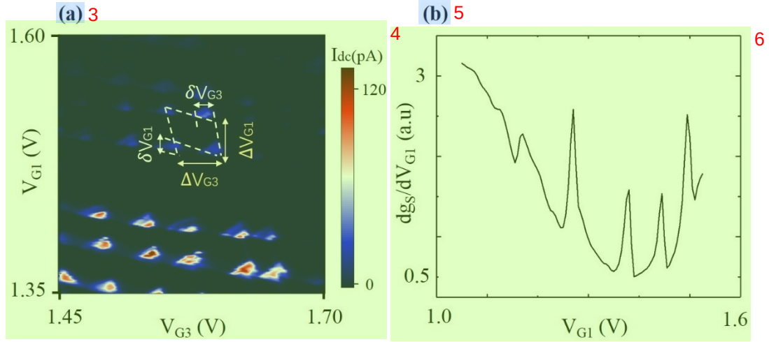
图 5.4(a) V_{SD} = 2 \text{ mV} , V_{G2} = 1.2 \text{ V} , 双量子点直流输运的电荷稳定性相图。(b) 空穴在双量子点之间输运时,会引起电荷感应器的电导变化从而观测到微分电导峰。 7
