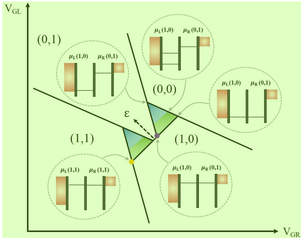
图 1.3 V_{SD} > 0 时两个空穴的双量子点电荷稳定性相图，图中观测到一组偏压三角形，4 虚线圆圈内插图为偏压三角形内部不同区域对应的量子点电化学势。
