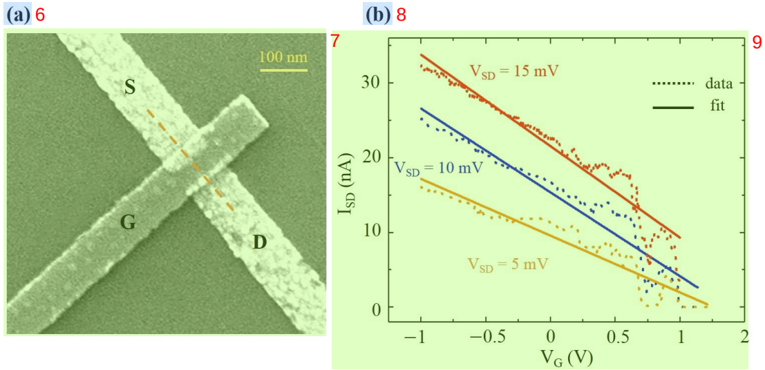
图 2.14 (a) Ge 纳米线场效应晶体管器件的 SEM 图，其中橙色虚线表示 Ge 纳米线。它和单量子点结构类似，包括源极 S、漏极 D、以及一个顶栅 G。(b) 不同 V_{SD} 下输运电流 I_{SD} 随顶栅电压 V_G 的变化曲线以及对应的线性拟合。
