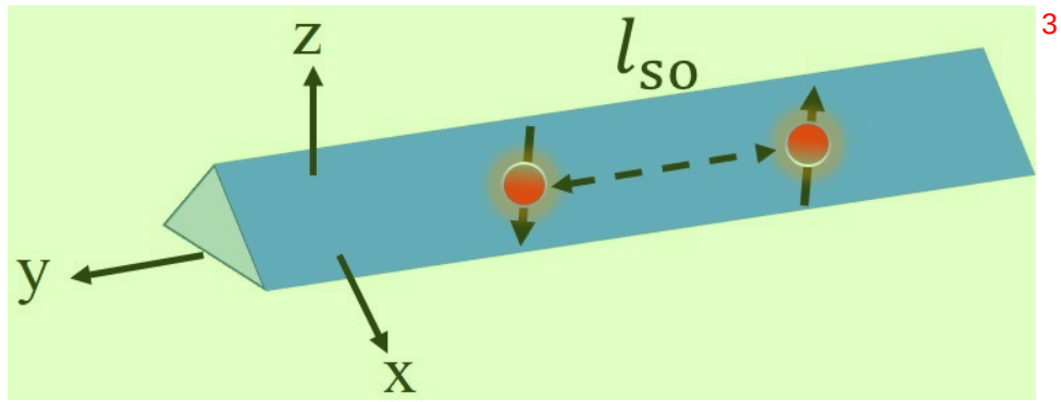
图 3.6 Ge 纳米线中自旋轨道耦合长度 l_{so} 示意图，外加磁场方向为 z 方向。 4
