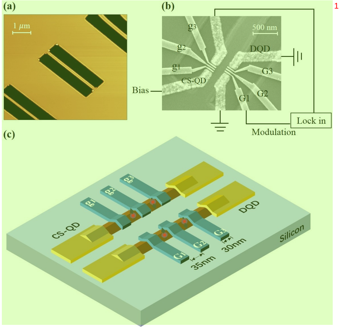
图 5.3 (a) 定位型 Ge 纳米线的原子力显微镜图，纳米线生长在硅图形衬底的沟槽边缘上。(b) 样品的扫描电子显微镜图，它由两个结构相同的双量子点构成，其中一个作为电荷感应器(CS-QD)。(c) 样品的三维立体结构示意图。
