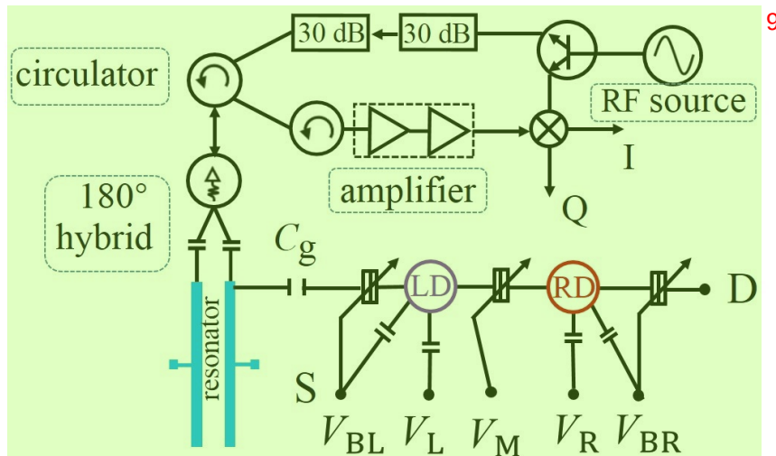
图 4.3 实验装置的等效电路示意图。 10
