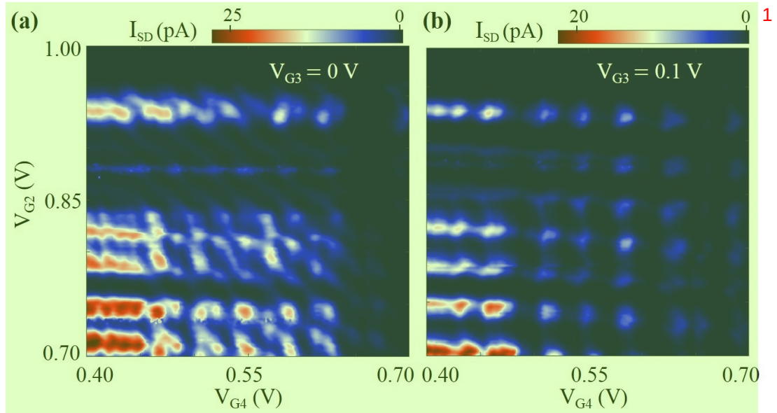
图 2.13 (a) V_{SD} = 0.5 mV, V_{G1} = V_{G5} = 0.5 V, V_{G3} = 0 V 时双量子点的蜂窝图。(b) 和(a) 相同区域但是在 V_{G3} = 0.1 V 下测量的双量子点相图。
