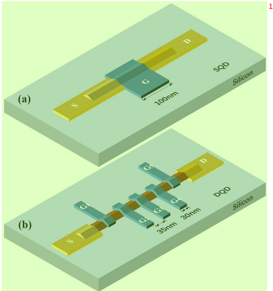
图 2.10 (a) 单量子点三维立体结构示意图。(b) 双量子点三维立体结构示意图。
