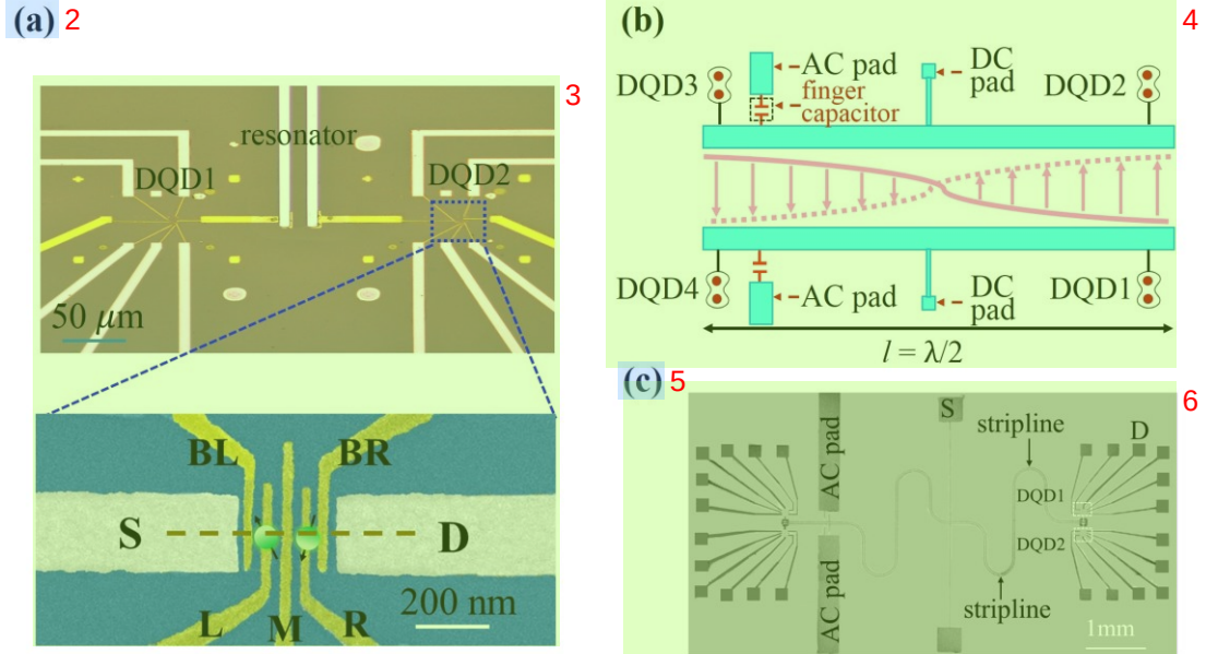
图 4.2 (a) 复合结构的光学显微镜图和 Ge 纳米线双量子点扫描电子显微镜图。双量子点 2 通过其源漏电极耦合到微波腔。 3 (b) 复合结构的示意图。半波长( \lambda/2 )微波腔的长度是 4 l = 12.5 \text{ mm} ，由两条超导带状线组成，通过交趾电容器耦合到微波输入和输出端口。两条带状线上的电势会产生相位相反的稳定电磁场。 5 (c) 复合结构的扫描电子显微镜图。 6
