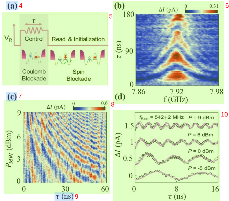
图 3.11 (a) 方波及脉冲序列图。(b) 外磁场 B = 100 mT, 功率 P = -15 dBm 时比特的 Rabi 振荡图。(c) 中心频率下，随功率变化的 Rabi 振荡图。(d) 选取 -5、0、6、9 dBm 下的振荡电流并拟合出 Rabi 频率。 11
