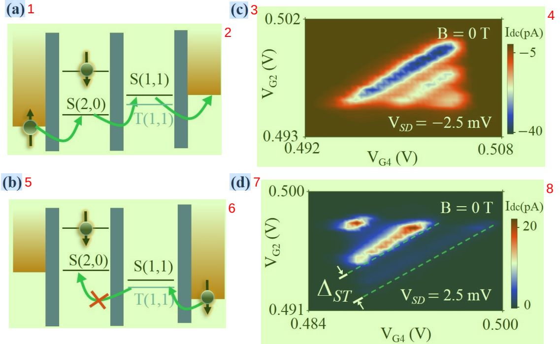
图 3.3 (a) 空穴在双量子点间运输的示意图，运输过程为 (1, 0) \rightarrow (2, 0) \rightarrow (1, 1) \rightarrow (1, 0) 。 (b) 源漏偏压方向相反时，由于泡利不相容原理，三重态 (1, 1) \rightarrow 单重态 (2, 0) 之间的运输被禁止。 (c) 当 V_{SD} = -2.5 \text{ mV} 时观测到的偏压三角形，运输过程对应于(a)。 (d) 当 V_{SD} = 2.5 \text{ mV} 时观测到的偏压三角形，运输过程对应于(b)。此时偏压三角形底部绿色虚线标注的区域电流被抑制，发生自旋阻塞。绿色虚线的间隔宽度对应于三重态 T(2, 0) 和单重态 S(2, 0) 之间的能级差 \Delta_{ST} 。
